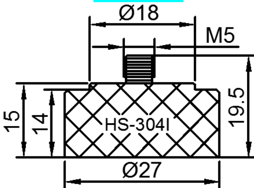
外形尺寸图
