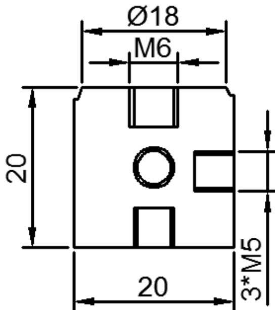
外形尺寸图
